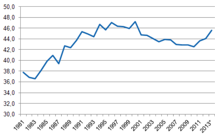
Figurbilaga 1. Skattekvoten, 1981–2013*
