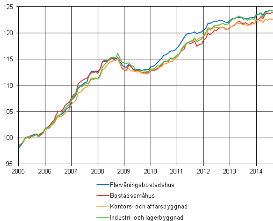
Figurbilaga 1. Byggnadskostnadsindex 2005=100
