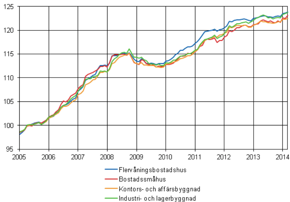
Figurbilaga 1. Byggnadskostnadsindex 2005=100
