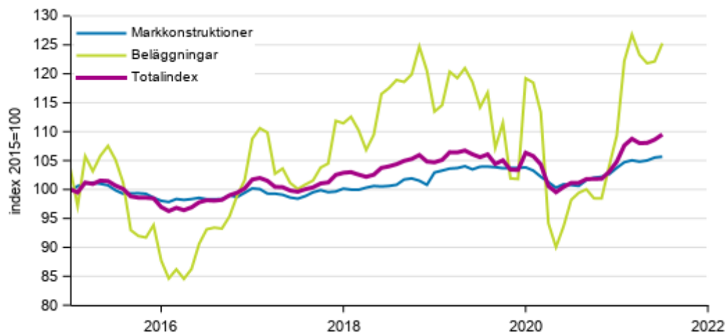
Figurbilaga 1. Kostnadsutvecklingen för Jordbyggnadsindexet (2015=100), totalindex, markkonstruktioner och beläggningar åren 1/2015–7/2021
